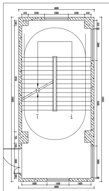
PLAN 高三西侧楼梯间2-5层平面图 比例: 1:38
