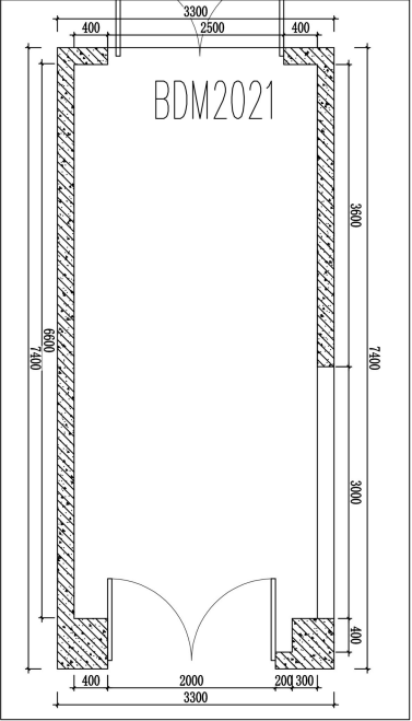
PLAN 实验楼一楼主原始平面图 比例 1:38
