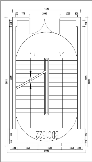
PLAN 实验楼楼梯间2-5层原始平面图 比例 1:38
