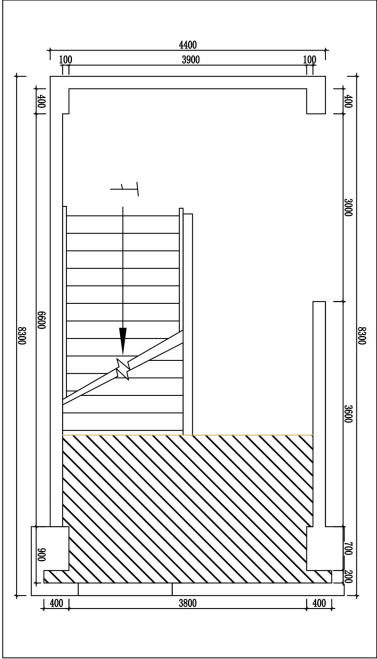
PLAN 实验楼楼梯间1层原始平面图 比例 1:38
