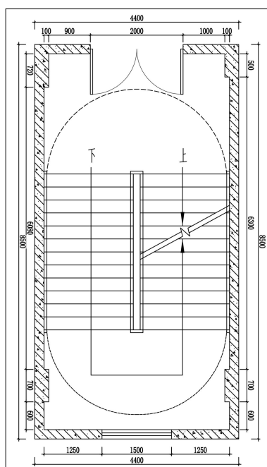
PLAN 高三东侧楼梯间2-5层平面图 比例: 1:38
