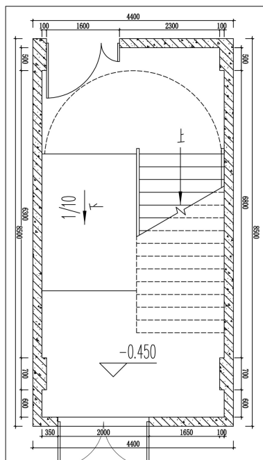
PLAN 高三东侧楼梯间1层平面图 比例: 1:38
