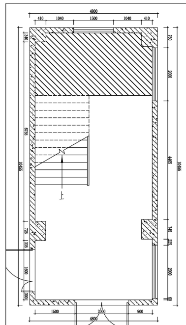
PLAN 高三西侧楼梯间1层平面图 比例: 1:38
