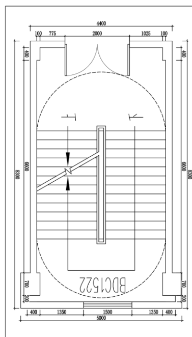
PLAN 实验楼楼梯间2-5层原始平面图 比例: 1:30
