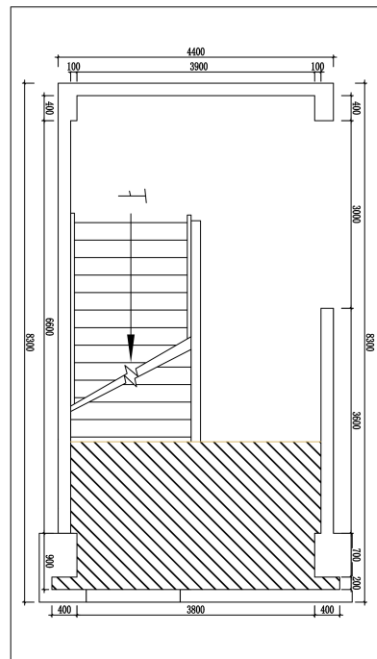
PLAN 实验楼楼梯间1层原始平面图 比例: 1:30
