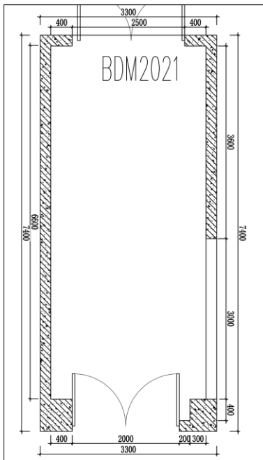
PLAN 实验楼一楼大厅原始平面图 比例: 1:30
