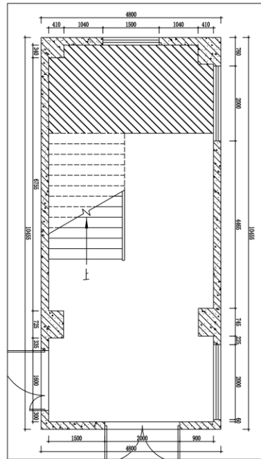
PLAN 高三西侧楼梯间1层平面图
