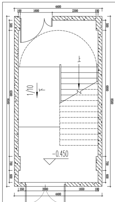
PLAN 高三东侧楼梯间1层平面图 比例: 1:35
