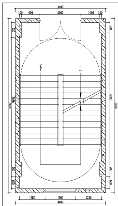
PLAN 高三东侧楼梯间2-5层平面图
