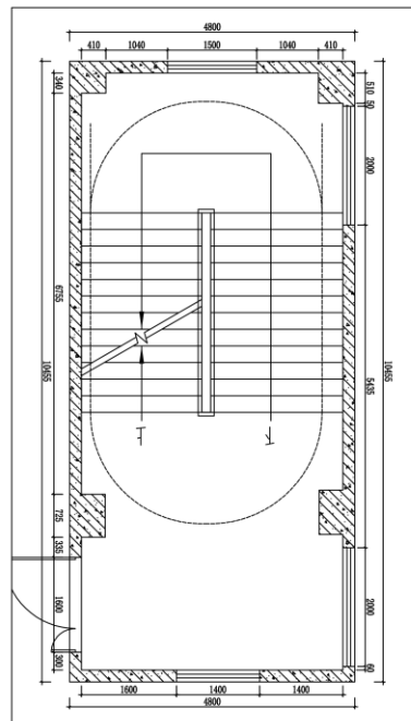
PLAN 高三西侧楼梯间2-5层平面图
