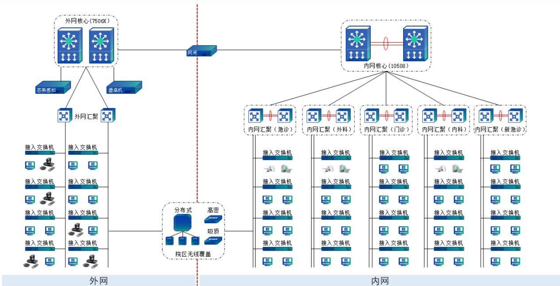
河南科技大学第一附属医院—景华院区接入网络架构图
