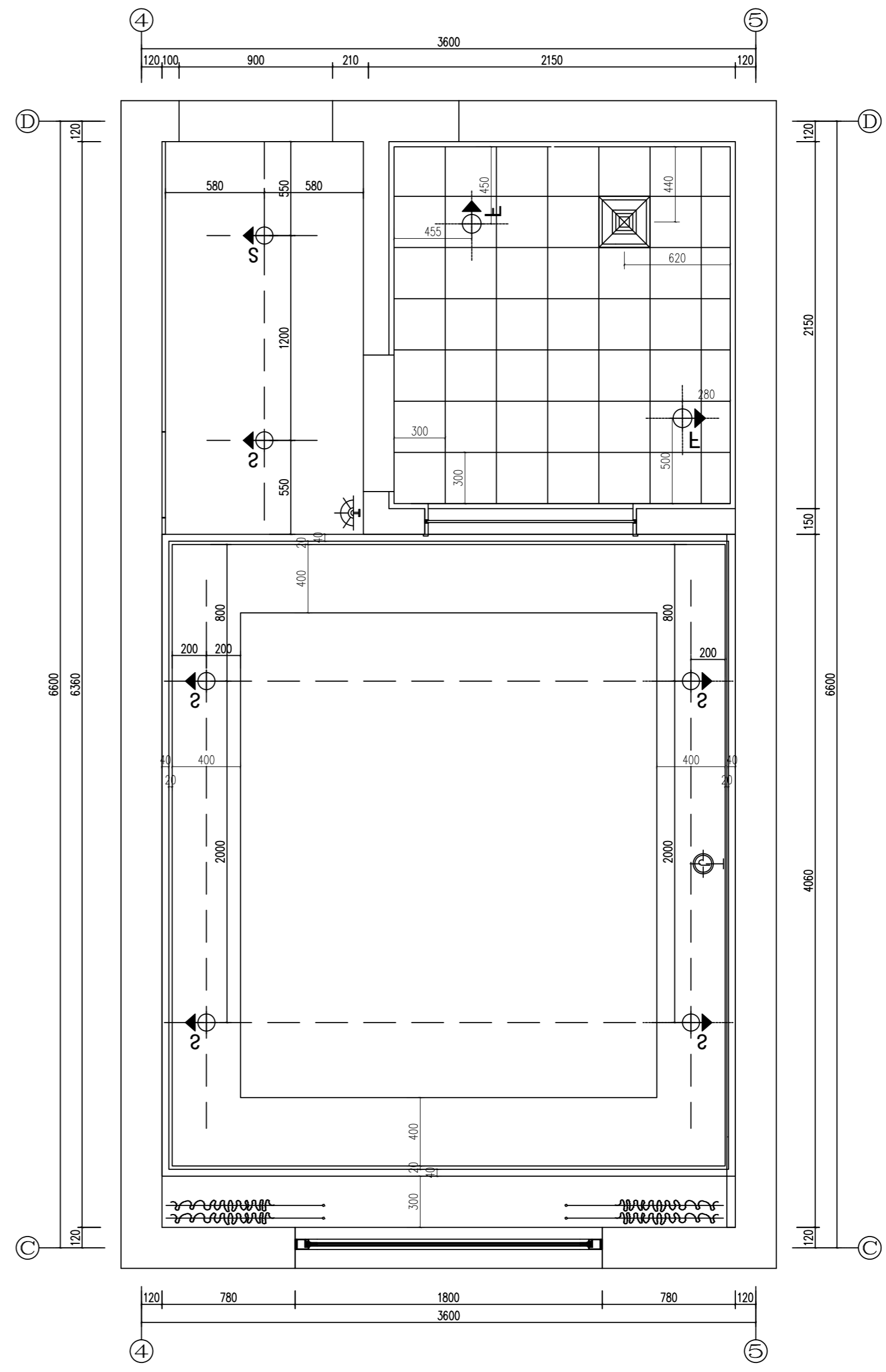
RC 平面图 3#楼双人宿舍天花尺寸及灯具定位图 Scale 1 : 25&A2
