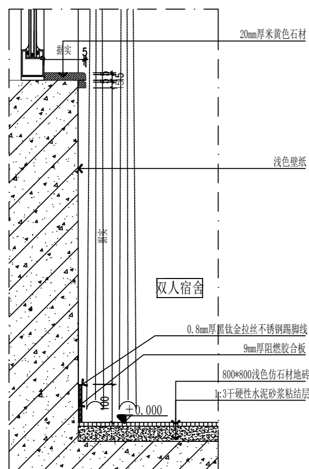
01 剖面图 窗台板剖面图 Scale 1 : 10&A2
