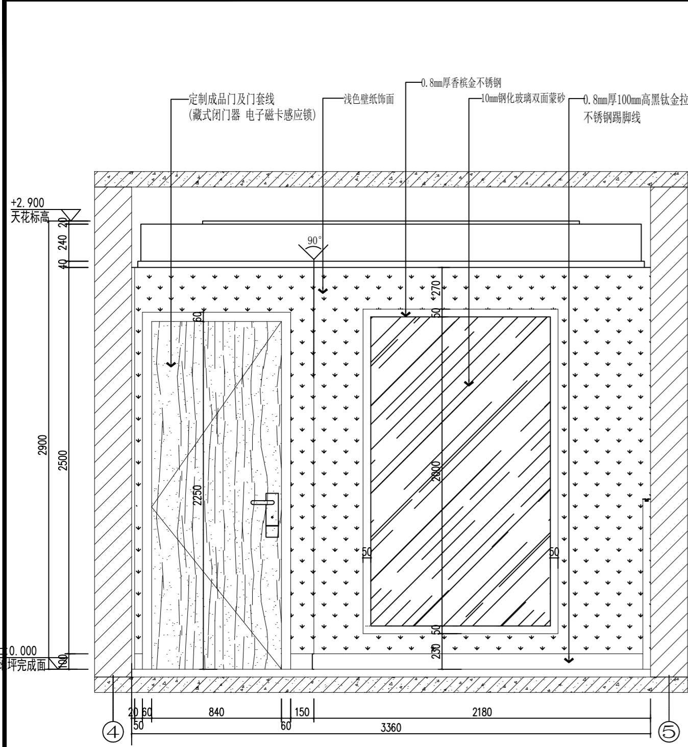
E1 立面图 3#楼双人宿舍立面图 比例 Scale 1 : 25&A2
