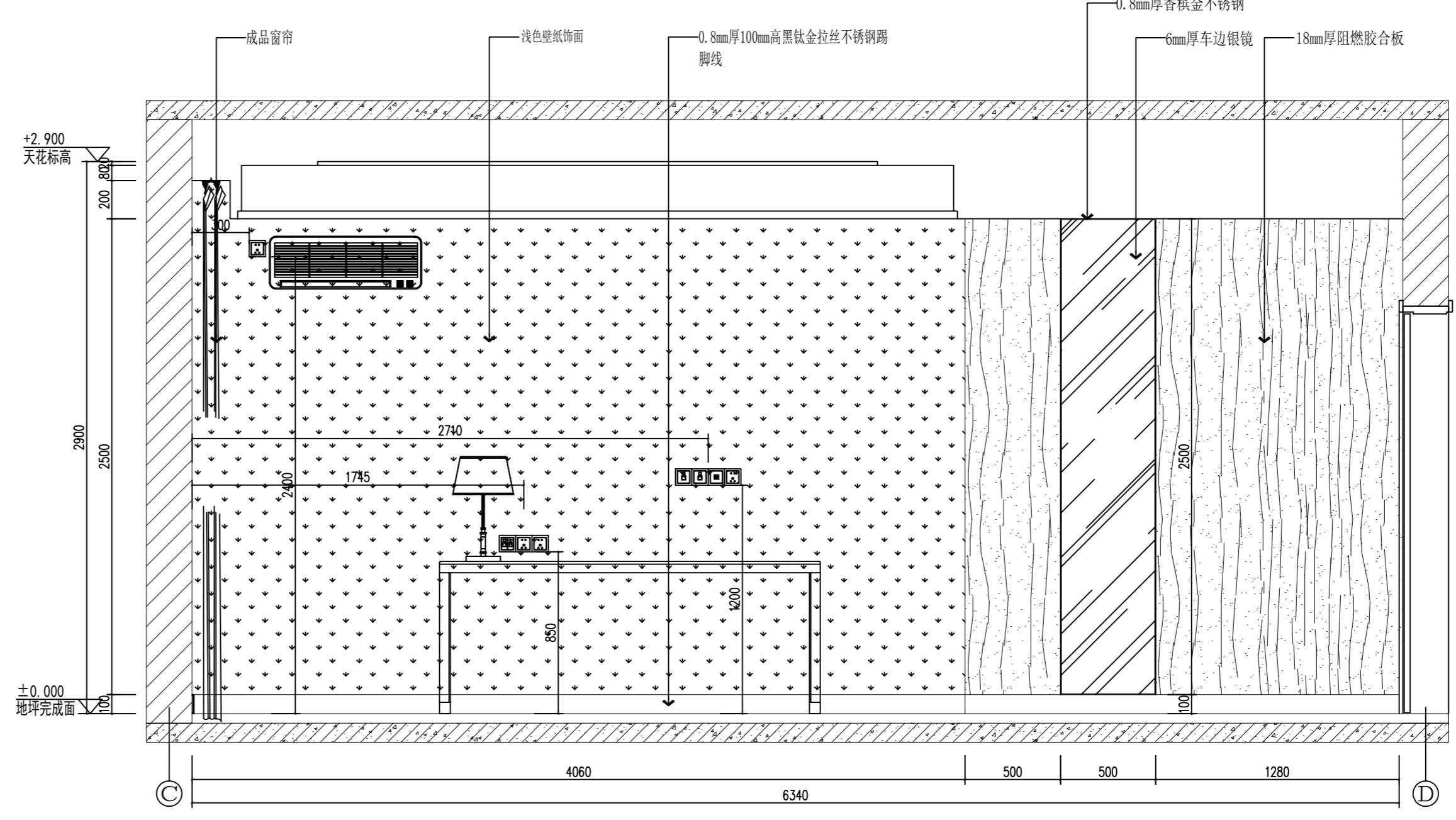
E4 立面图 3#楼双人宿舍立面图 比例 Scale 1 : 25&A2
