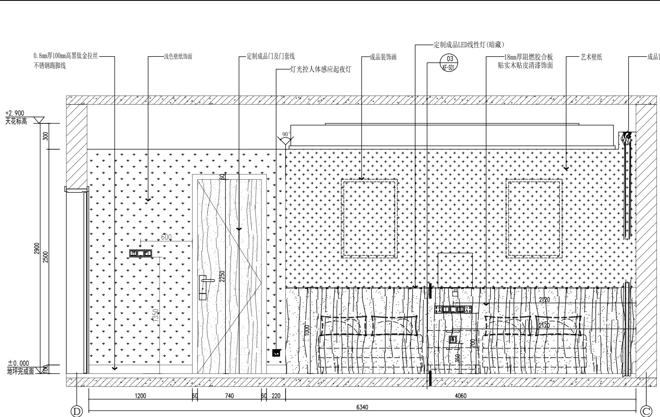
E2 立面图 3#楼双人宿舍立面图 比例 Scale 1 : 25&A2
