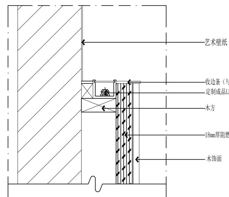
03 剖面图 背景墙节点图 KF-E01 Scale 1 : 2&A2
