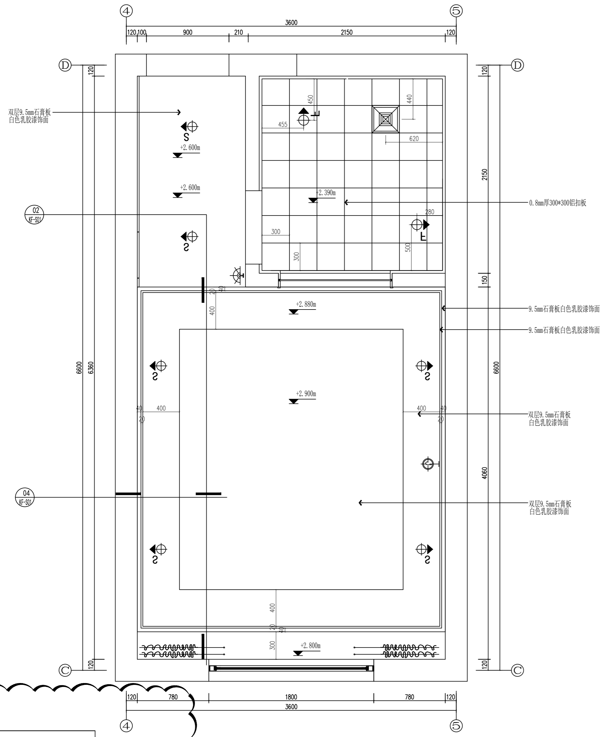
RC 平面图 3#楼双人宿舍天花吊顶图 Scale 1 : 25&A2
