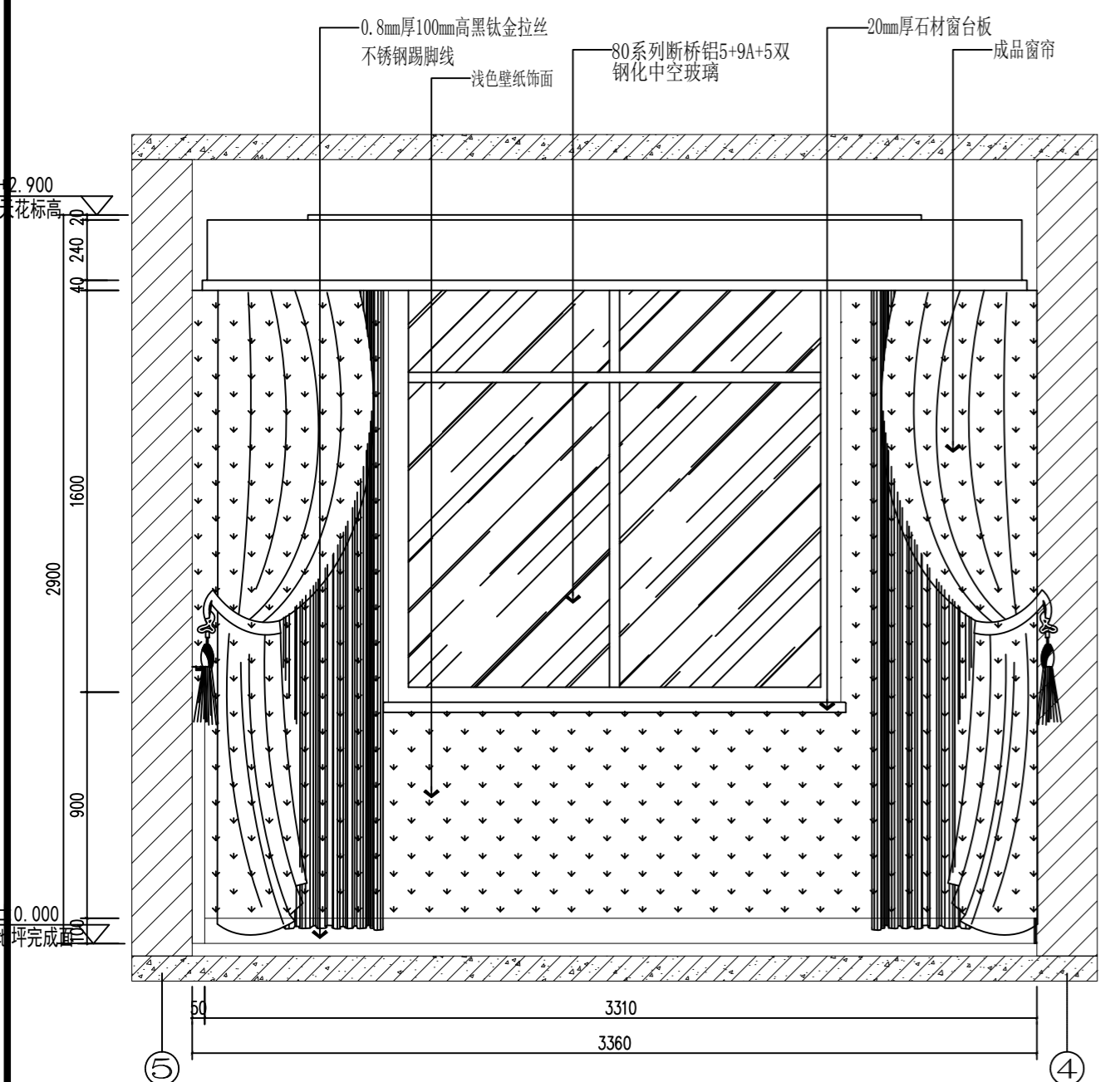
E3 立面图 3#楼双人宿舍立面图 比例 Scale 1 : 25&A2
