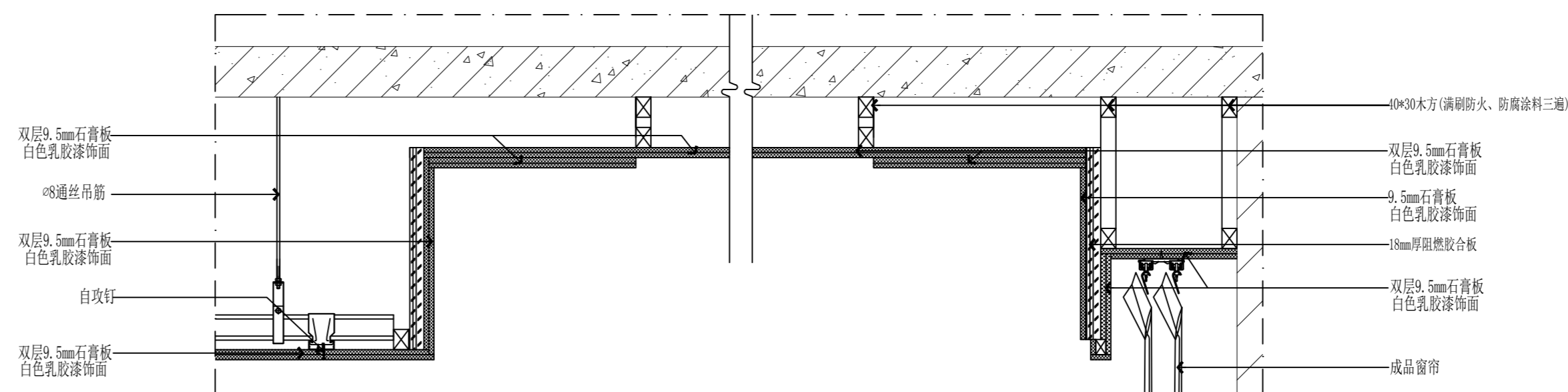
02 剖面图 双人宿舍天花节点图 KF-P02 Scale 1 : 10&A2
