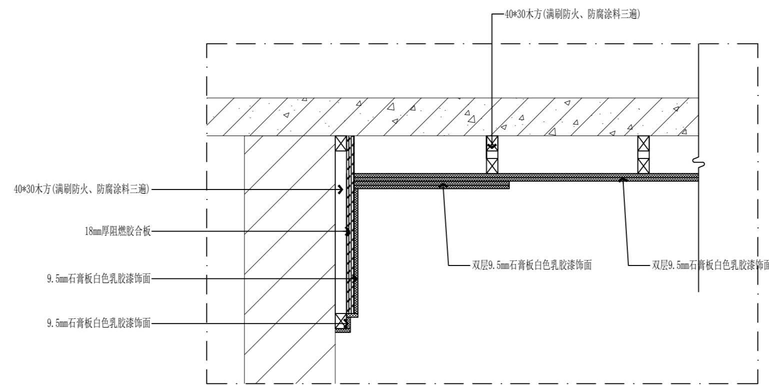
04 剖面图 双人宿舍天花节点图 KF-P02 Scale 1 : 10&A2
